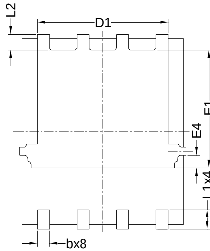
Bottom View 背面视图
